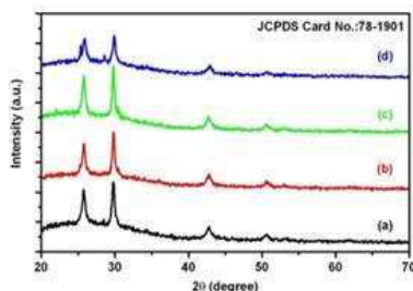
Fig. 1. XRD patterns of PbS thin films for deposition time i.e. a) 20 min, b) 30 min, c) 40 min, and d) 50 min.
